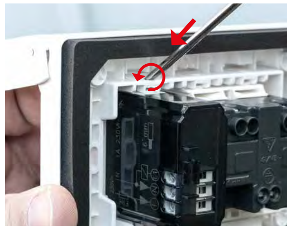
Devices coupling and removal from the rear part ربط الأجهزة وإزالتها من الجزء الخلفي
